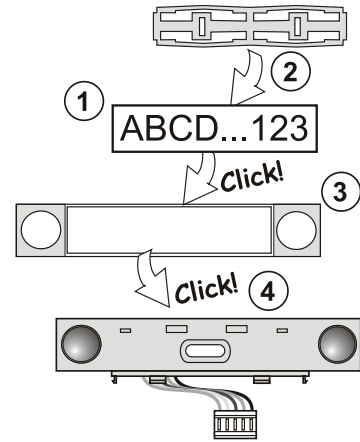
Bild: Einlegen des Beschriftungsschildes ins Bedienungsegment.
