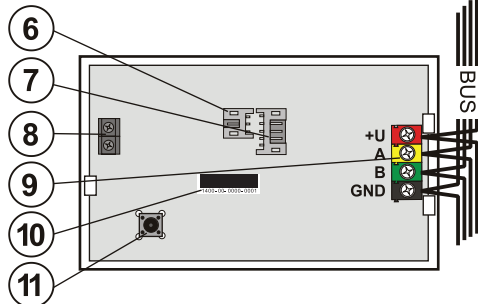
Bild: 6 – Stecker für den Anschluss des Audiomoduls; 7 – Stecker für die Bedienungsegmente; 8 – Klemmleiste für die Verbindung des Audiomoduls mit der Zentrale; 9 – Bus- Klemmleiste; 10 – Seriennummer; 11 – Sabotageschalter
